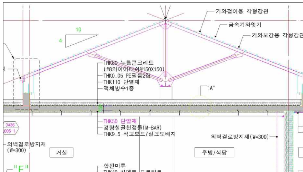
[그림 5] ♡♡♡♡ S-1블록 최상층세대 천정 단열재 설치 도면
